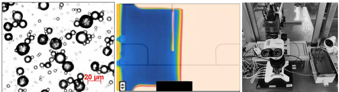
Abbildung 1: v.l.n.r.: Schmelzemulsion mit unterkühlten und kristallisierten Tropfen; beispielhafte Wärmebildaufnahme eines Mikrofluidikchips zur Untersuchung der Kontaktkristallisation; Versuchsaufbau.
