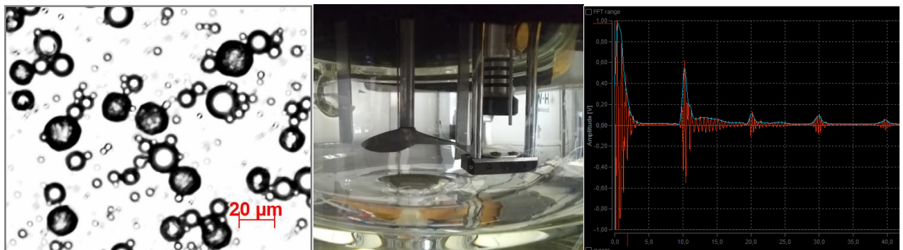
Abbildung 1: v.l.n.r.: Schmelzemulsion mit unterkühlten und kristallisierten Tropfen; Blick in den 1L-Rührkessel; beispielhaftes Ultraschall-Signal einer n-Hexadecan-in-Wasser Emulsion mit dem Emulgator Tween®20.
